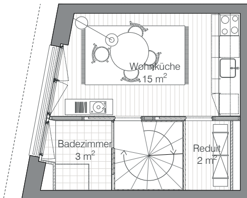
1. Obergeschoss
